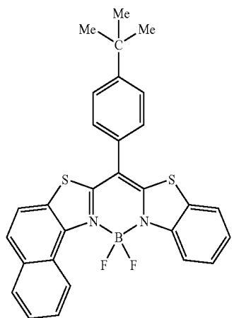
DHMB 2
