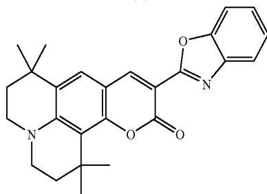
C-525T
