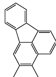
2,3-FlAn
