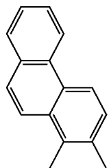
1,1-PhAn
