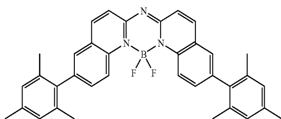
Blue 2
