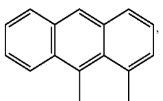
1,9-An
