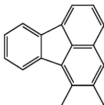
1,2-FlAn
