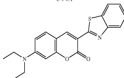
C-6
