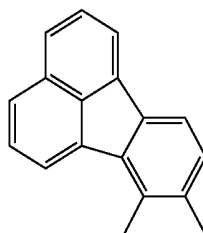
7,8-FlAn
