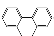
2,2'-BP
