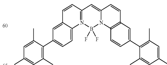
DPMB 1
