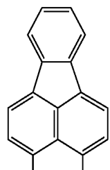
1,2-Pyr
