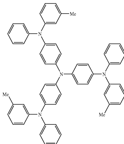
mTDATA:
